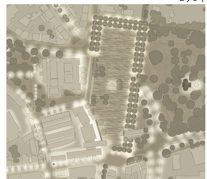
beleuchtungskonzept m 1:1000
